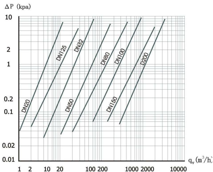
压力损曲线
