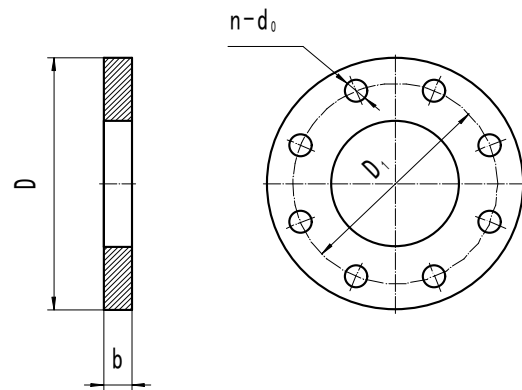
连接法兰
