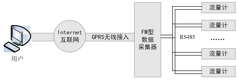
GPRS 无线接入的因特网传输
